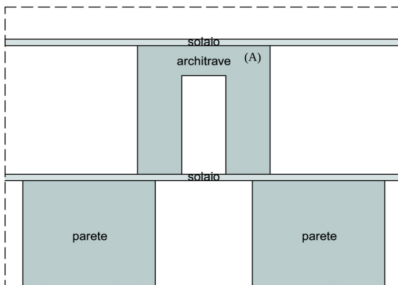
Figura 13: Parete con apertura (porta).
