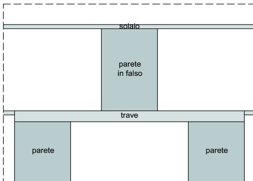
Figura 15: Parete in falso su trave.
