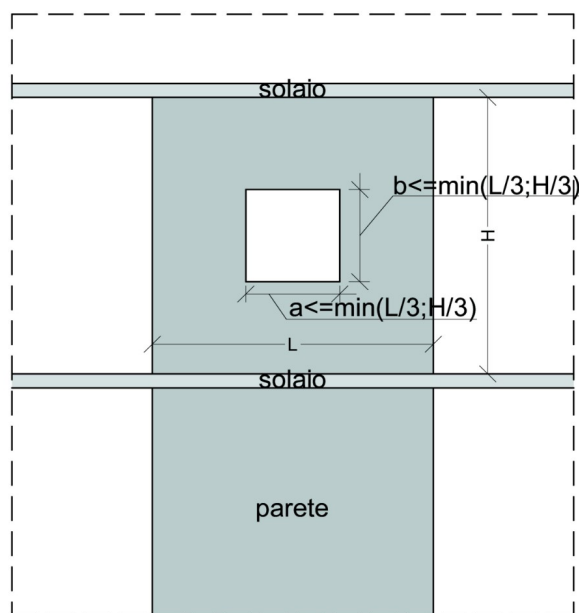
Figura 9: Parete con piccola apertura (finestra).
