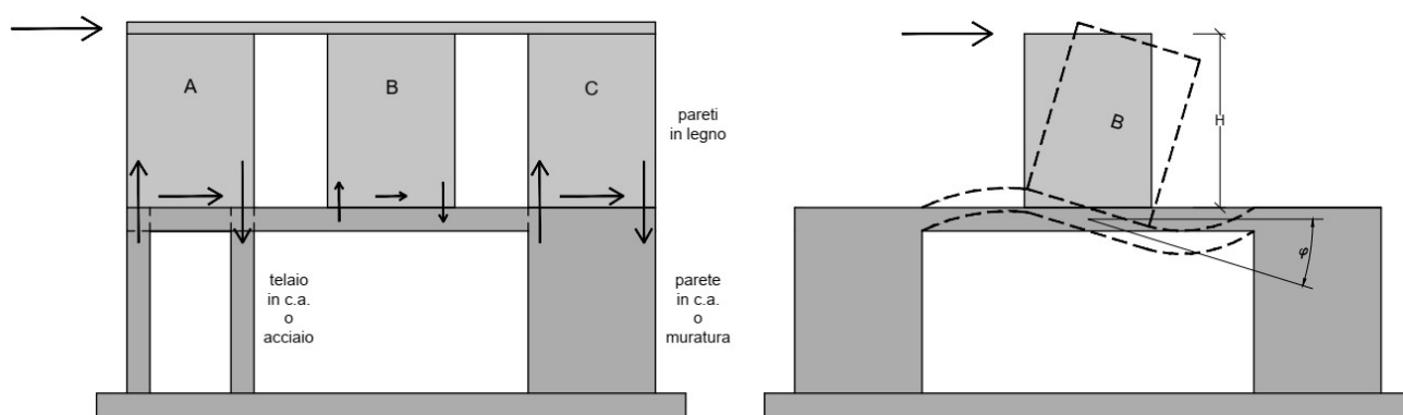
Figura 17: Le pareti di legno A e C poggiano su supporti rigidi (pareti in c.a. o muratura, telai in c.a. o acciaio). La parete B poggia su di una trave; la sua deformabilità alle azioni orizzontali è determinata non solo dalla deformabilità dei pannelli e delle unioni ma c'è anche l'importante contributo dato dalla deformabilità alla rotazione della sottostante trave.
