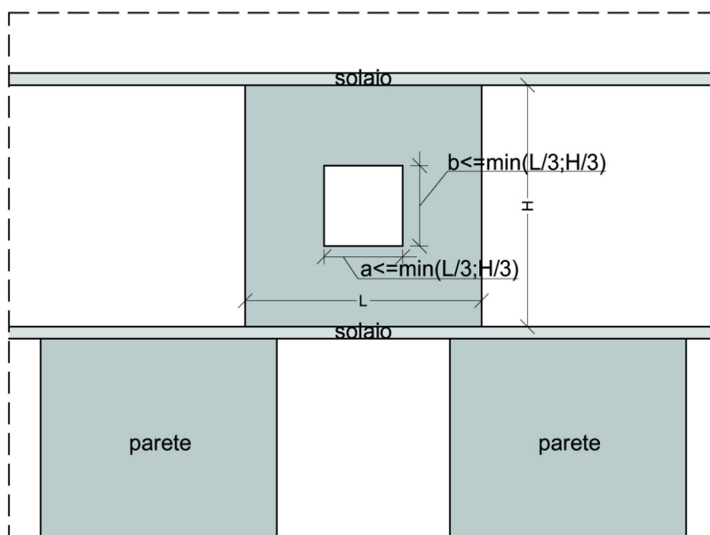
Figura 12: Parete con piccola apertura (finestra).
